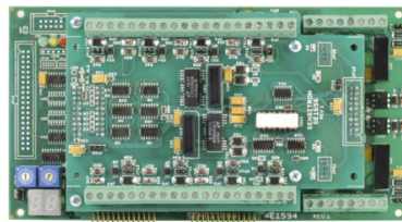
Modulo ingressi analogici AIM Analog Inputs Module AIM
